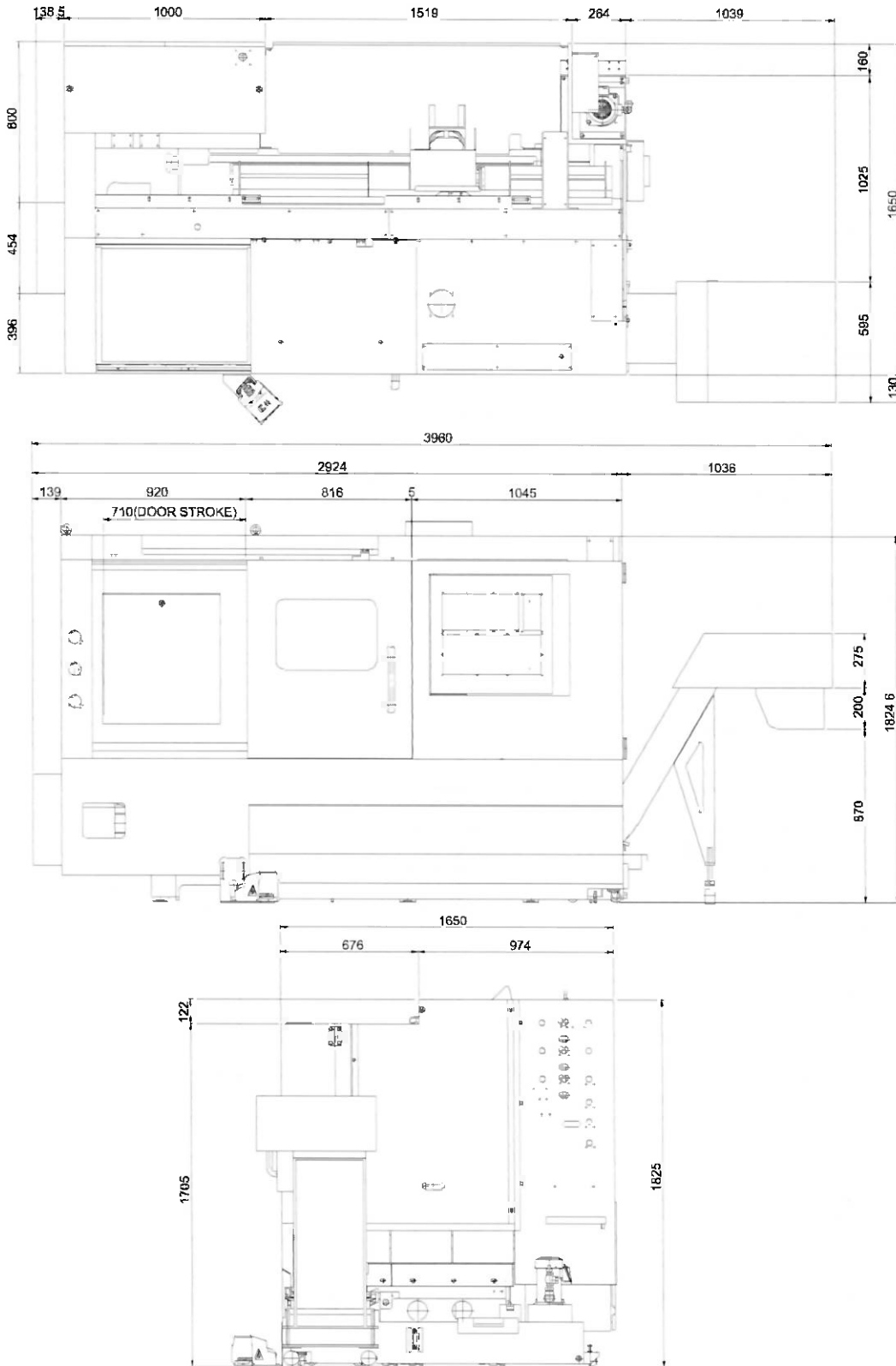
그림 1.4 외형 치수도 (단위: mm)
